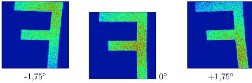
Abbildung 9: Abbildungsänderung bei Verdrehung des Scannerspiegels
